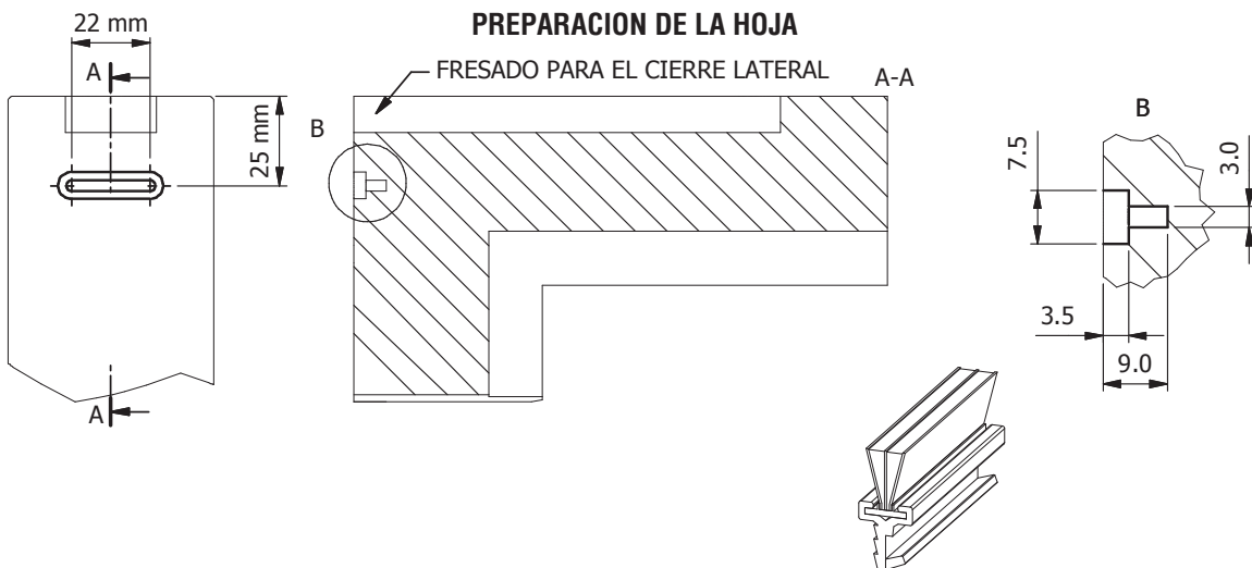
Trocito de burlete con soporte incorporado Ref; UK688N/G-1000
