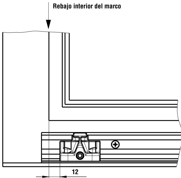
Montaje del tope con muelle
