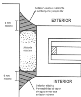
Figura 22. Sellado a testa
