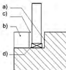
Figura 25. Definición de un galce de acristalamiento
