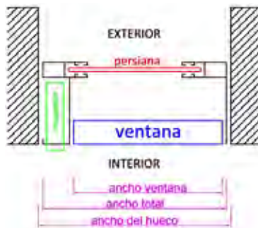
Figura 46. Esquema sección horizontal de ventana con persiana y recogedor a la izquierda embutido en guía, con solución asimétrica y muro de cerramiento de gran espesor
