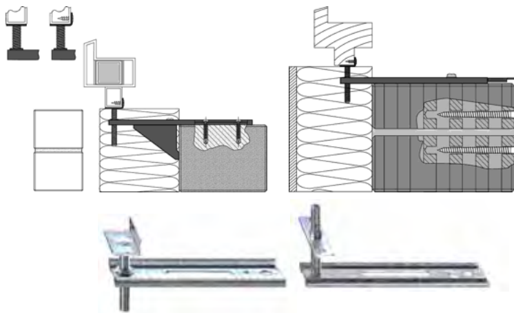
Figura 20. Consolas
