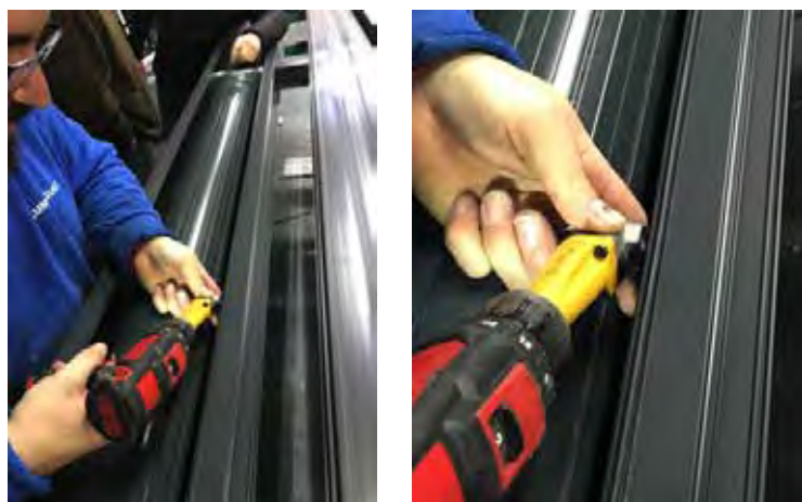
Figura 61. Atornillado del cajón a la ventana
