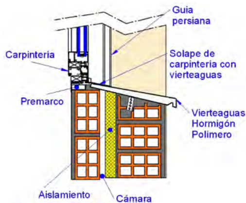
Figura 85. Esquema vierteaguas
