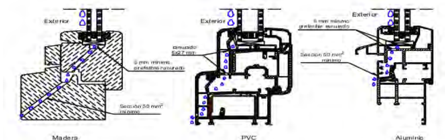
Figura 24. Ejemplos ilustrativos de sistemas de drenaje
