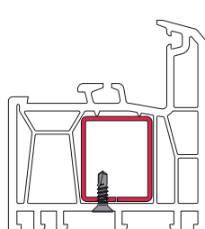
Tornillo Tipo 1
