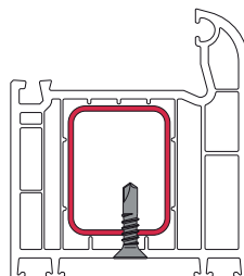
Tornillo Tipo 2
